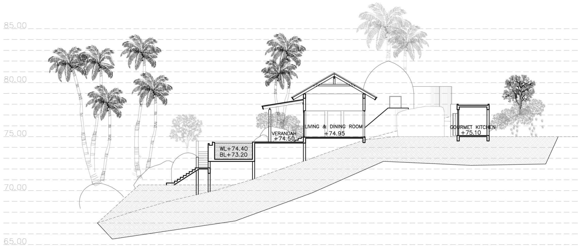
SECTION B VILLA : PLOT 4
