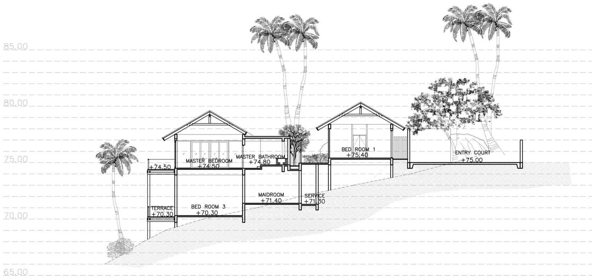
SECTION A VILLA : PLOT 4
